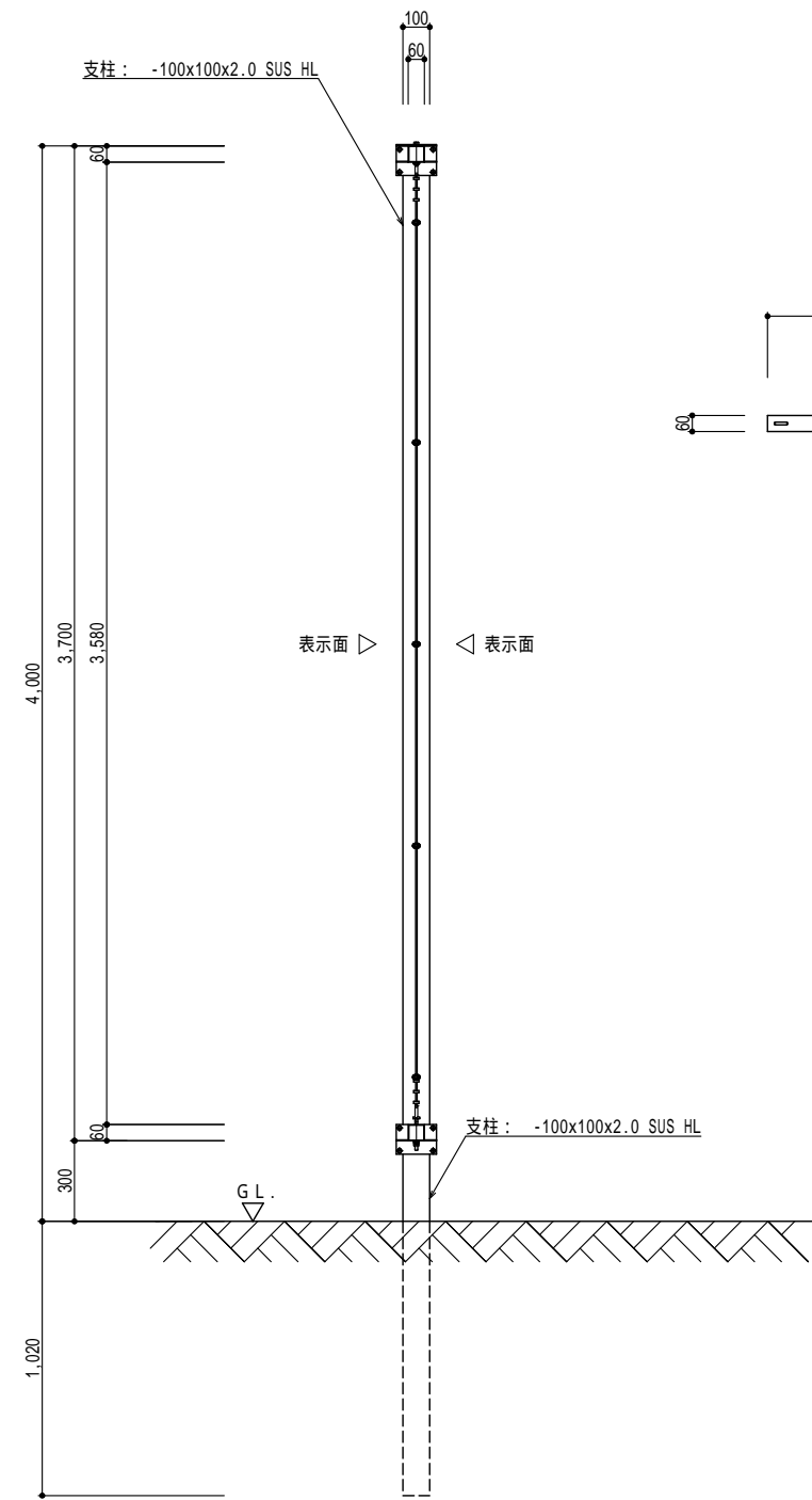
側面図 S=1/30
