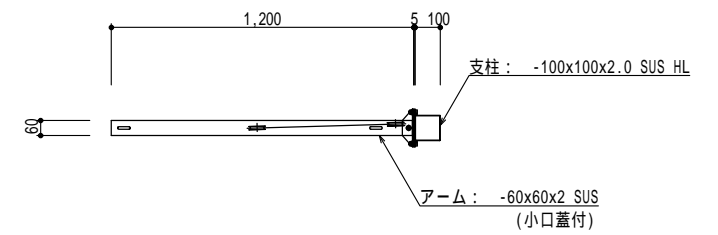
平面図 S=1/30
