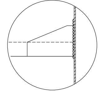
角鋼管に取付の場合 B 現場 4面溶接
