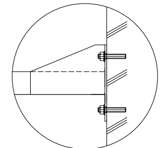
壁面に取付の場合 アンカーボルト (別途)
