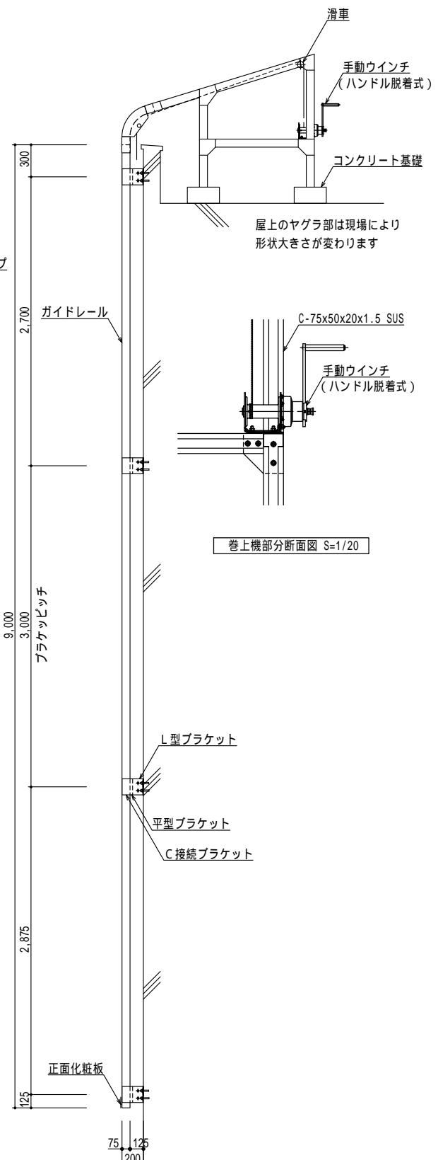
側面図 S=1/50
