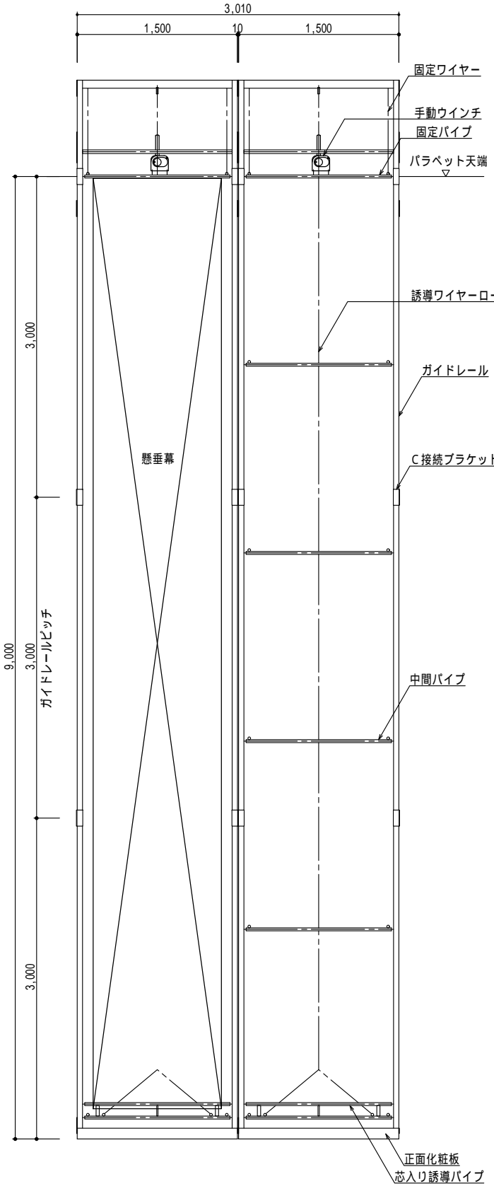
正面図 S=1/50
