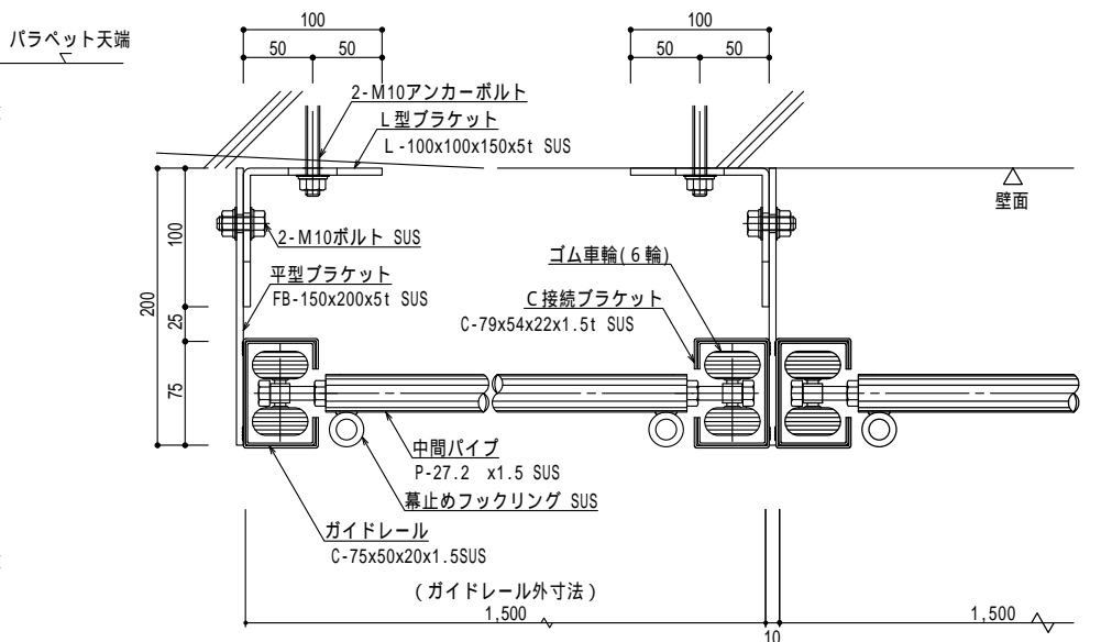
平面断面図 S=1/6
