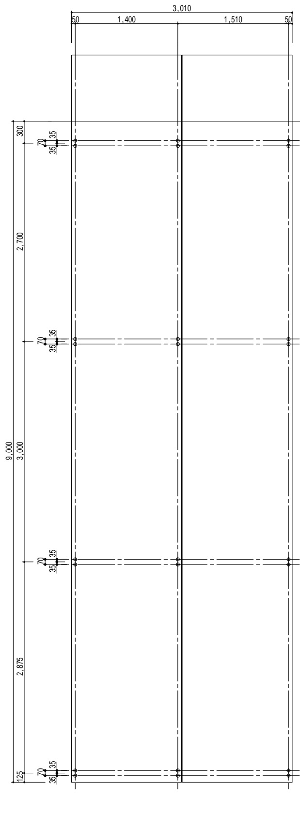
アンカー位置図 S=1/50
